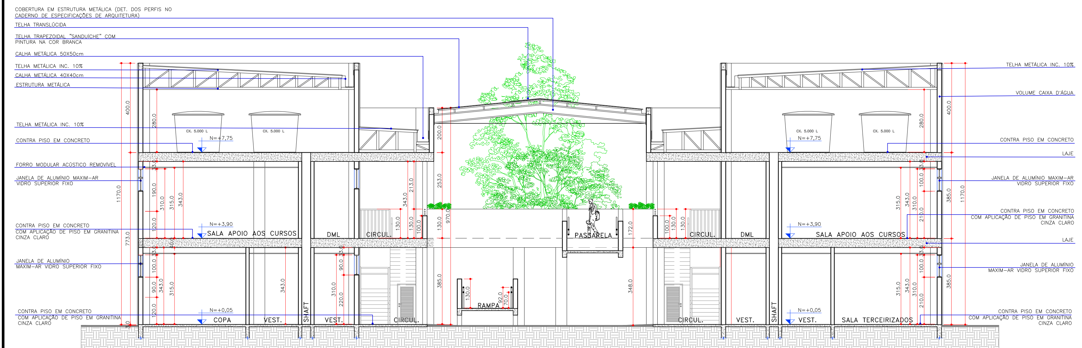
CORTE T1 ESC. 1/100
