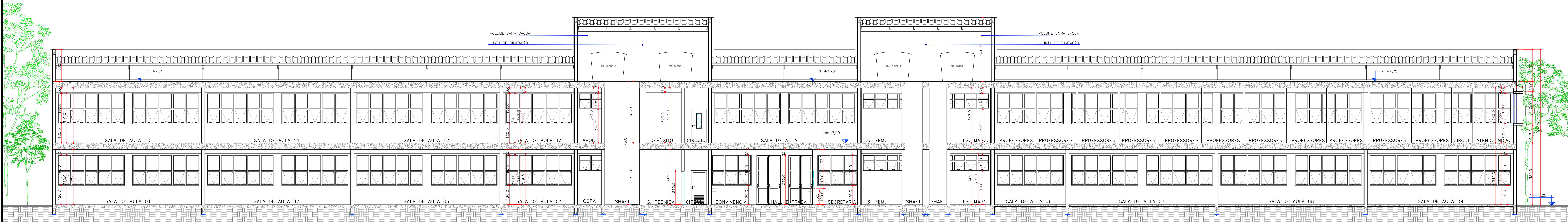
CORTE L3 ESC. 1/100
