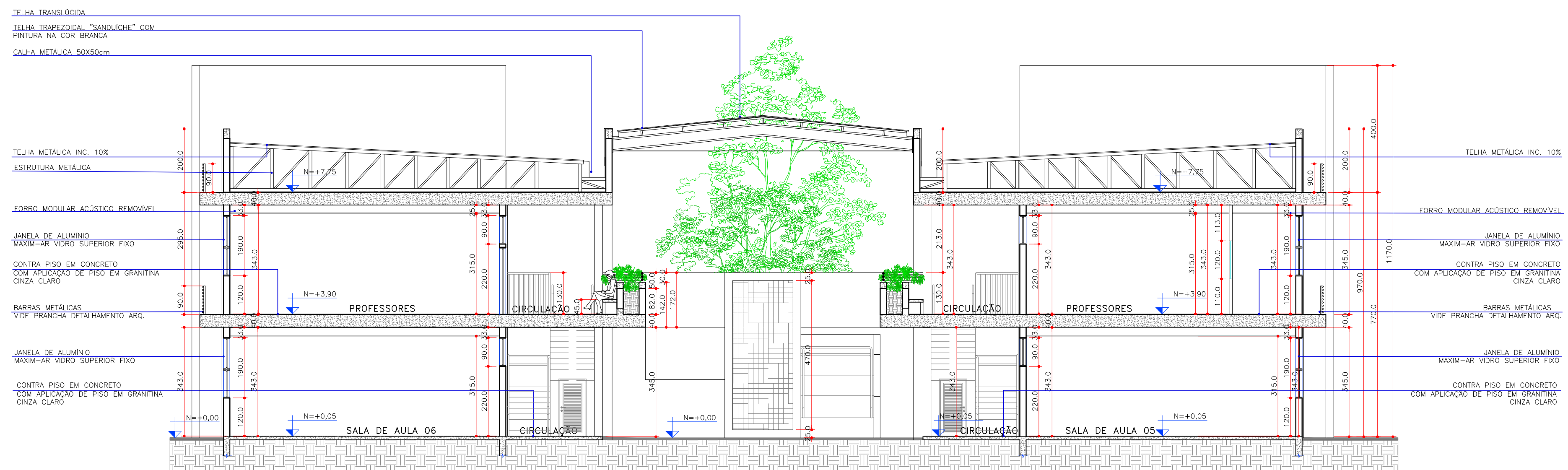
CORTE T2 ESC. 1/100
