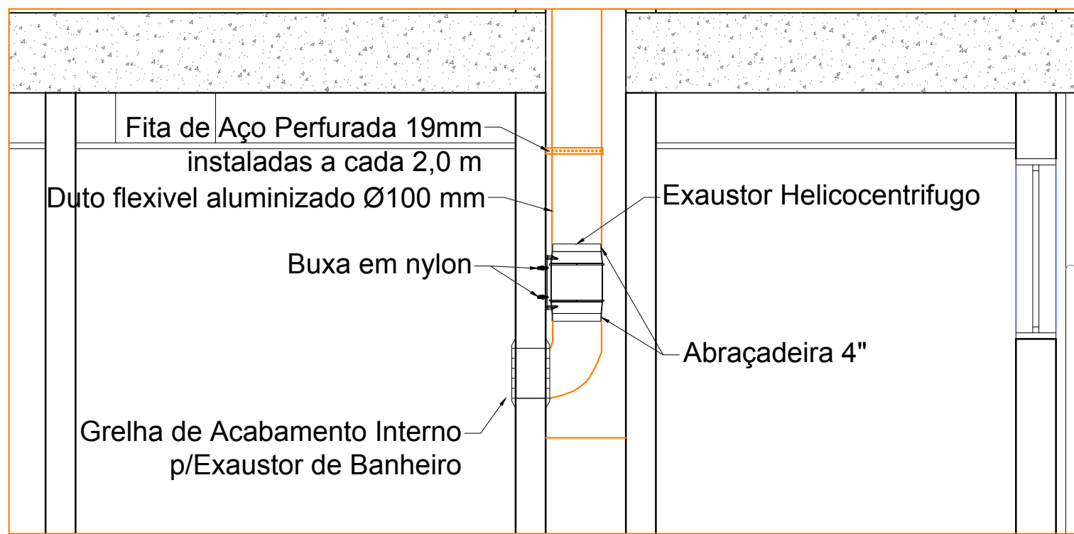
DETALHE A Sem Esc.
