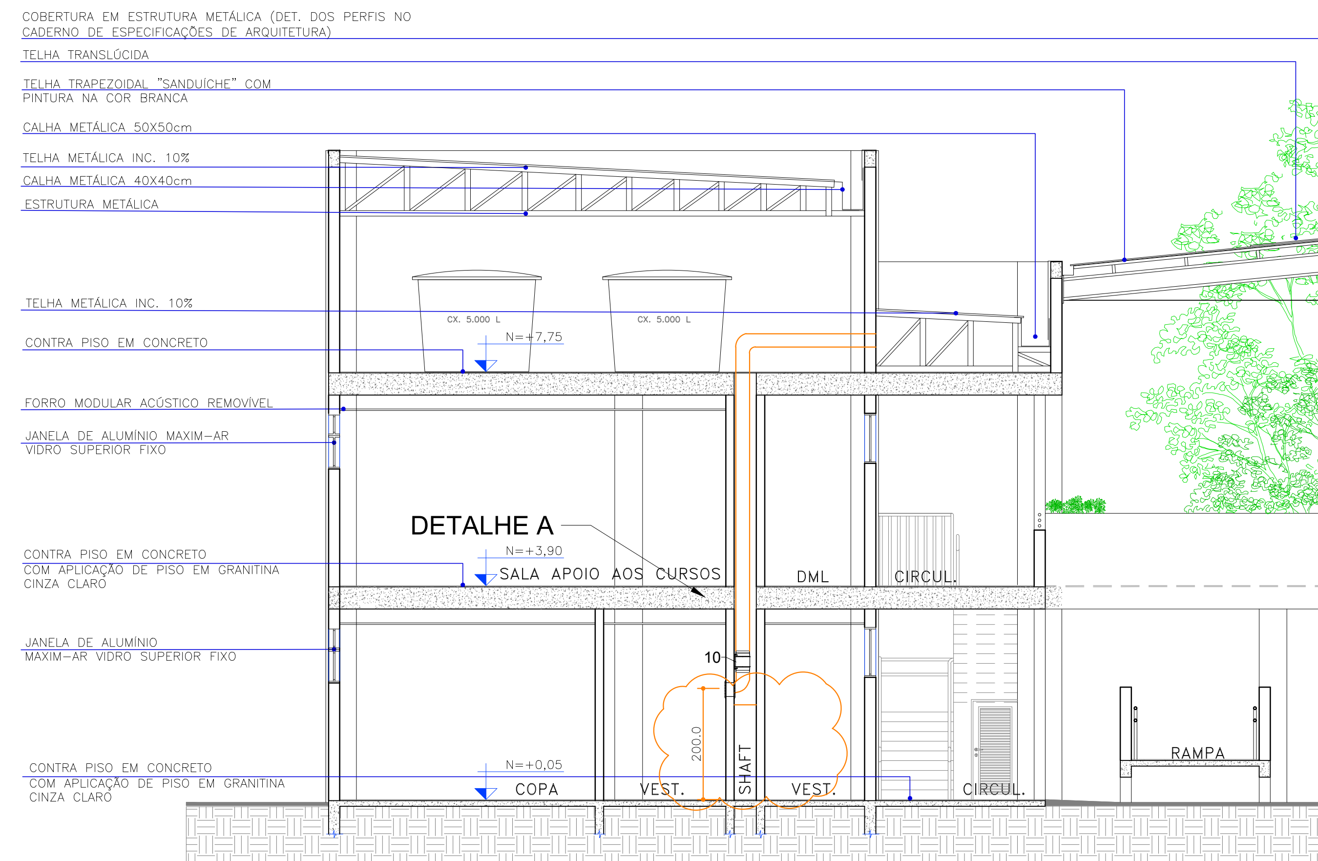
CORTE T1 Sem Esc.
